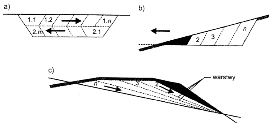
Rys. 5. Metody prowadzenia wykopów
