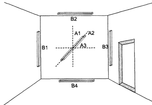
Rys.2. Sprawdzenie odchylenia od płaszczyzny i krawędzi A1 - pionowe ustawienie łąty, A2 - ukośne ustawienie łąty ~ 45°, A3 - poziome ustawienie łąty, B1 i B3 - poziome ustawienie łąty na przeciwległych krawędziach ściany, B2 i B4 - poziome ustawienie łąty na przeciwległych krawędziach
